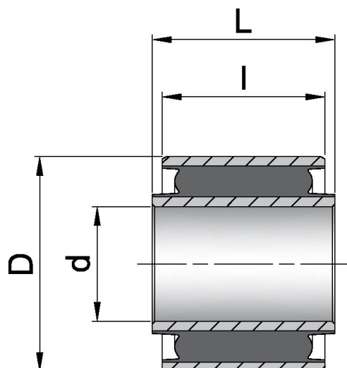
TOLLERANZE DIAMETRO INTERNO (d) INSIDE DIAMETER (d) TOLERANCES
